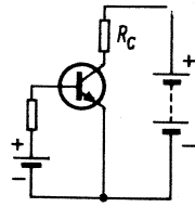
Bild 11. Erzeugen der Basisspannung durch eine Batterie
