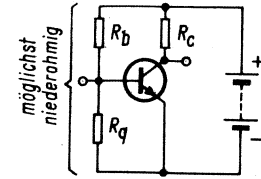
Bild 12. Basisspannung durch Spannungsteiler erzeugt
