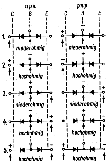
Bild 20. Richtwirkung der Elektrodenübergänge
