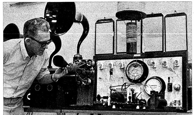
Bild 1. Der erste Telefoniesender von Poulsen in Laboratoriumsausführung. In der Mitte die Flammenkammer mit Rohren für die Wasserstoffversorgung, davor eine Spule des magnetischen Gebläses, links das unmittelbar in die Antenne geschaltete Siebenfach-Kohlemikrofon
