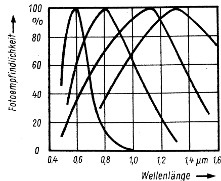
Kurven von Chalkogeniden-Gläsern unterschiedlicher Zusammensetzung. Durch Wahl der Glas-sorten läßt sich die maximale Fotoempfindlichkeit für bestimmte Längenwellenbereiche erzielen
