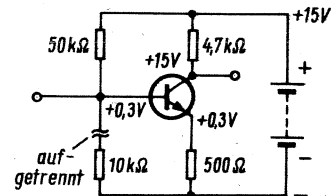
Bild 17. Spannungen an den Elektroden bei kurzgeschlossener Basis-Emitter-Strecke
