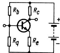
Bild 13. Stabilisierung der Basisspannung durch Stromgegenkopplung
