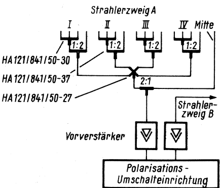
Bild 5. Schematische Darstellung der VHF-Empfangsantenne gemäß Bild 4. Bei Programmsteuerbetrieb sind alle 17 Kreuzdipole eingeschaltet. Die innere Antenne wird über den Zweifachhauptverteiler HA 121/841/50-37, die mittleren Strahler über den Vierfachverteiler HA 121/841/50-27 und die äußeren Strahler über den Vierfach- und den Dreifachverteiler HA 121/841/50-30. Daraus ergeben sich die angestrebten Amplitudenverhältnisse 1 : 0,58 : 0,24
