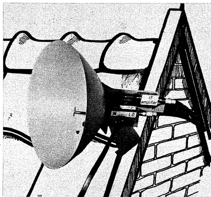
Bild 3. Modell einer 12-GHz-Empfangsanlage mit Parabolantenne und direkt ammontiertem Umsetzer mit Schottky-Barrier-Diode im Oszillator. Die Anlage ist eine Gemeinschaftsentwicklung der Philips-Laboratorien in Holland, Großbritannien und der Bundesrepublik
