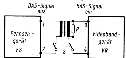
Bild 1. Prinzipschaltung der Videoauskopplung
