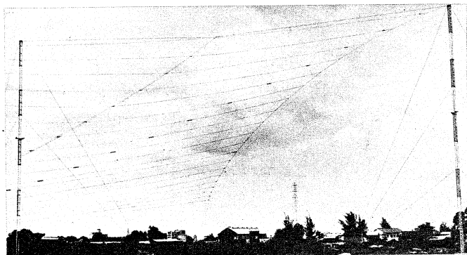
Diese 31 m hohe Richtantenne in Darassalam (Tansania) ist ausschließlich mit Parafilseilen verspannt. Aufgrund der Dehnungsfestigkeit ist ein Nachspannen kaum erforderlich (Werkaufnahme: ICI Faser-Vertriebsgesellschaft mbH)
