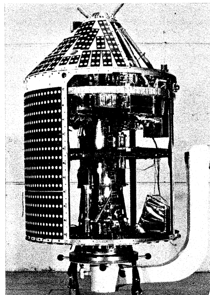
Bild 1. Der erste deutsche Forschungssatellit Azur auf dem Prüfstand
