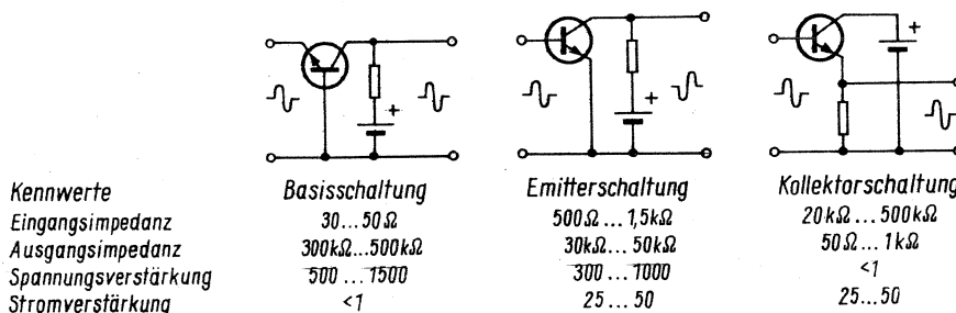
Bild 6. Grundschaltungen und Kennwerte als Verstärker
