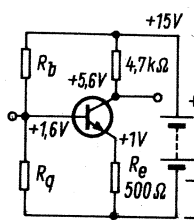
Bild 14. Verstärkerstufen mit Germanium-pnp-Transistor (a) und Silizium-npn-Transistor (b)
