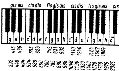
Tonfrequenzen der schwebenden Stimmung bezogen auf Kammerton \bar{a} = 440 Hz Halbtonverhältnis 1 : 1,059 \Delta \approx 6\%
