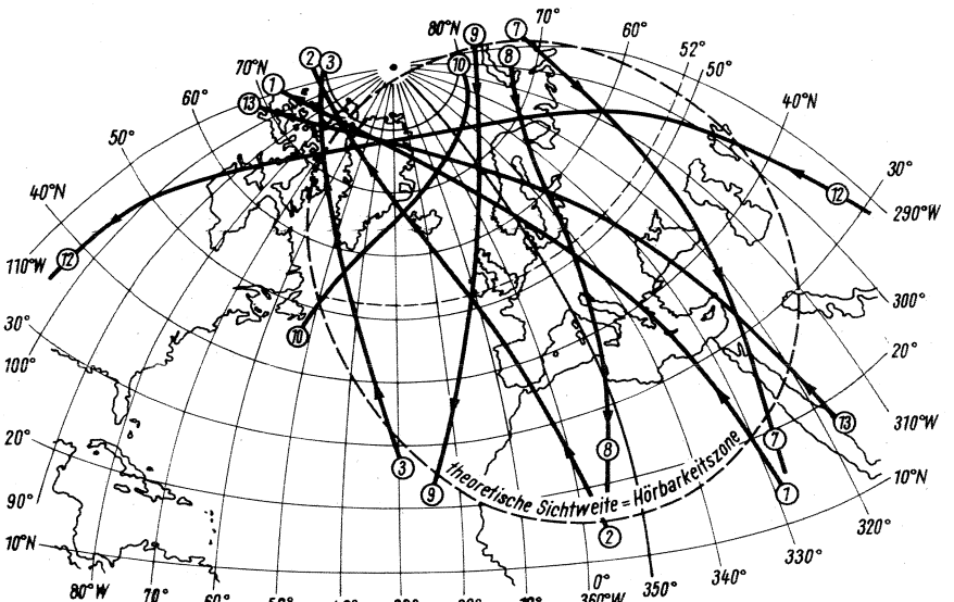
Bild 1. Errechnete Oscar-Bahndaten. Die Zahlen nennen die Umläufe, nicht aufgeführte sind nicht hörbar
