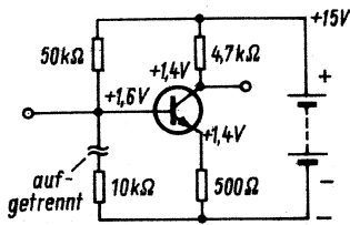
Bild 19. Spannungen an den Elektroden bei kurzgeschlossener Emitter-Kollektor-Strecke
